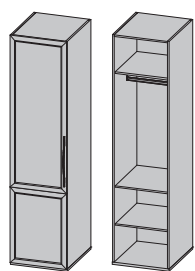
Шкаф со штангой (левый) С 101-лв 2191x540x615
